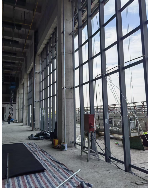
六、室内柱面龙骨
