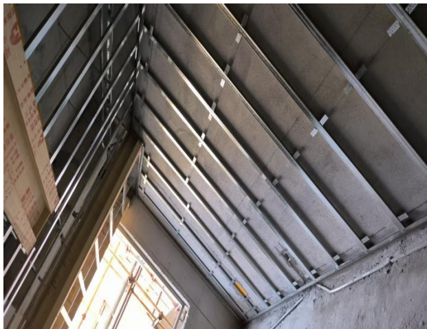
六、吊顶石膏板安装
