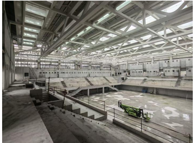
六、屋面不锈钢天沟安装
